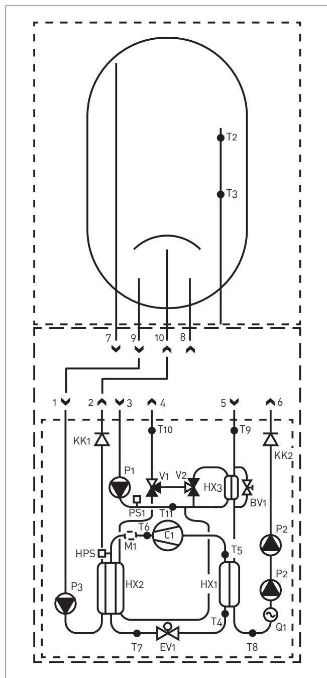
Warmtepomp WPU-KC 5G + Onderomkasting WPU + voorraadvat WPV
